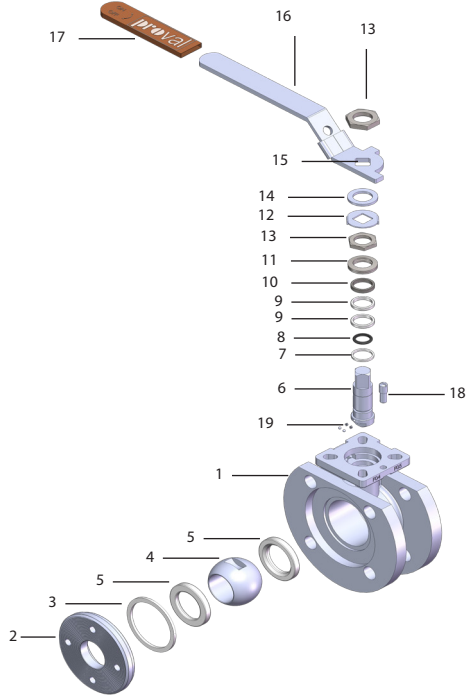
ISO5211 Top Flange
